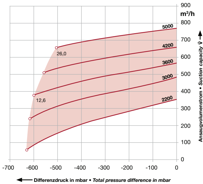
2BH2 0540 dreistufig · triple stage
