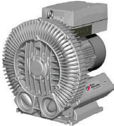
Seitenkanalverdichter G-BH2 e mit integriertem FU Side channel blower G-BH2 e with integrated FC
