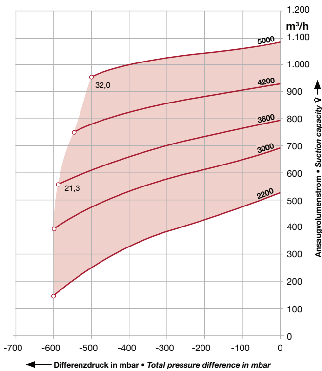
2BH2 0780 dreistufig · triple stage
