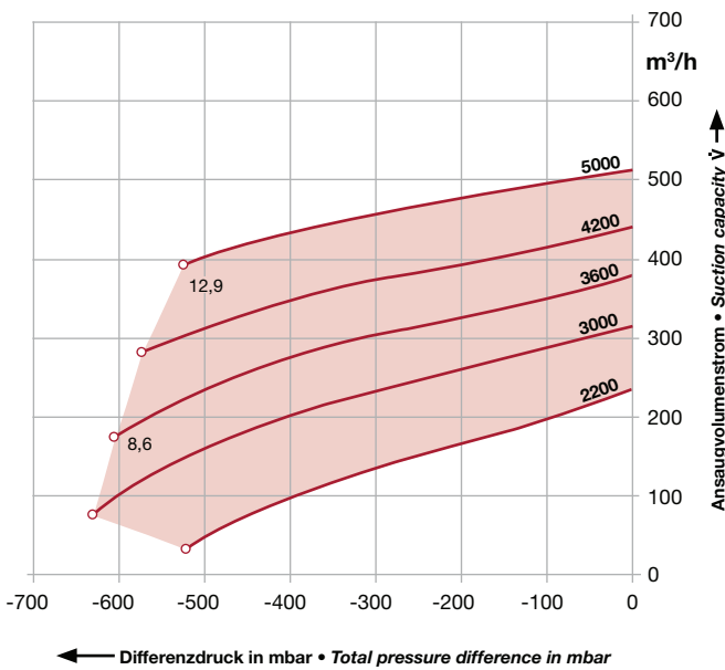
2BH2 0360 dreistufig · triple stage
