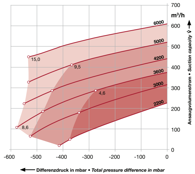
2BH2 0360 zweistufig · double stage
