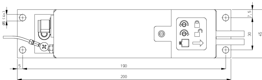
Technische Zeichnung CMME
