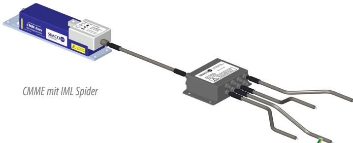
Abnehmbare Hochspannungsverteilerblock
